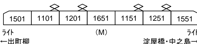
編成図 A9990
