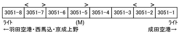
編成図 A6474
